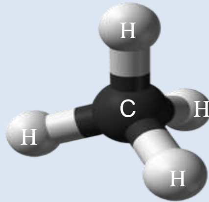
Метан CH 4
